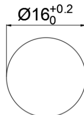
安装孔图
