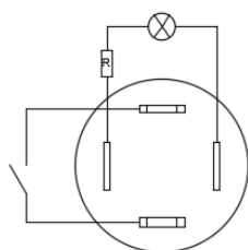
电器简图
