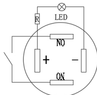
电气简图
