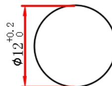
安装孔图
