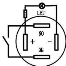
电气简图
