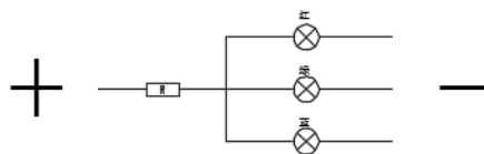
电气简图
