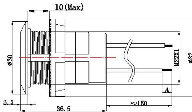
安装孔图
