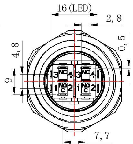
安装孔图
