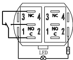
电气简图
