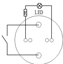
电气简图
