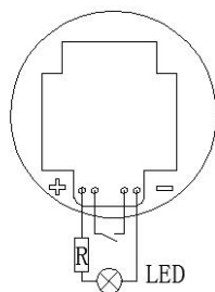
电气简图
