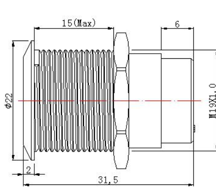
安装孔图
