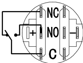
电气简图
