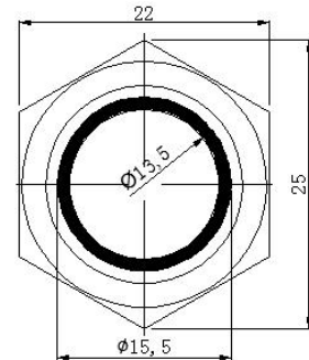
安装孔图
