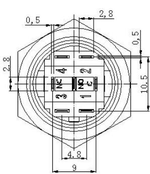
电气简图
