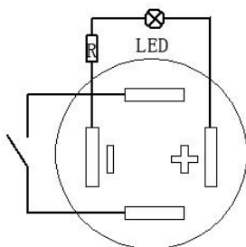
电气简图
