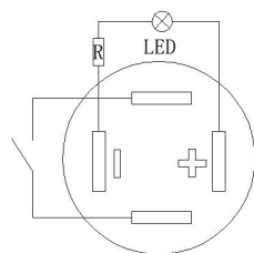
电气简图
