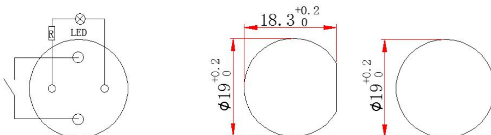
电气简图
