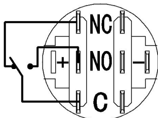
电气简图
