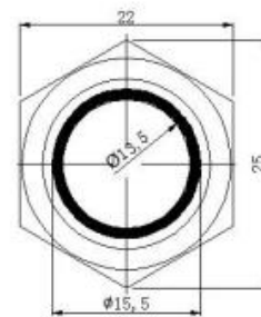
安装孔图
