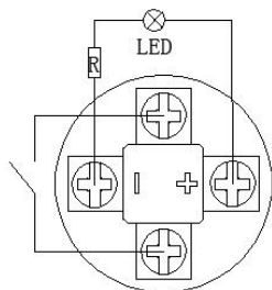
电气简图
