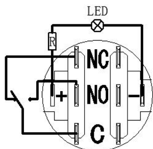
电气简图
