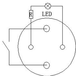
电气简图
