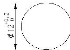
安装孔图
