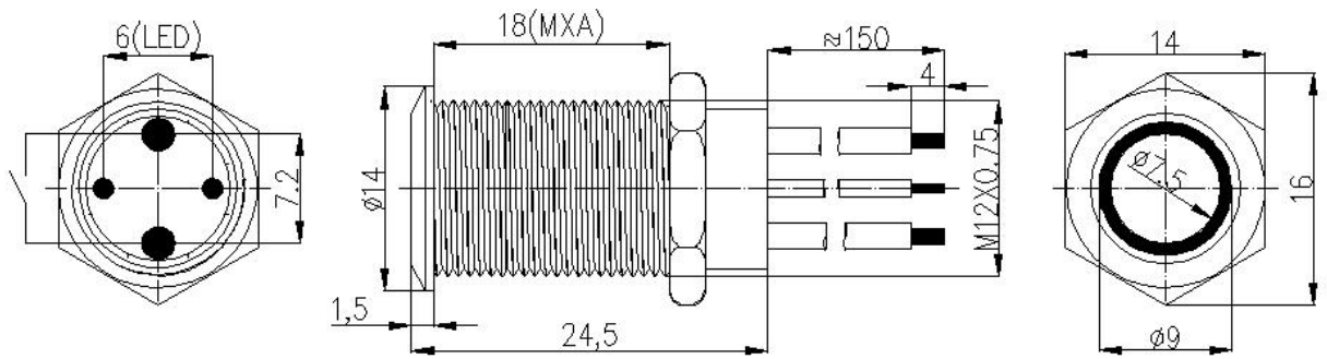
安装孔图
