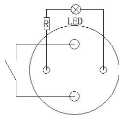
电气简图
